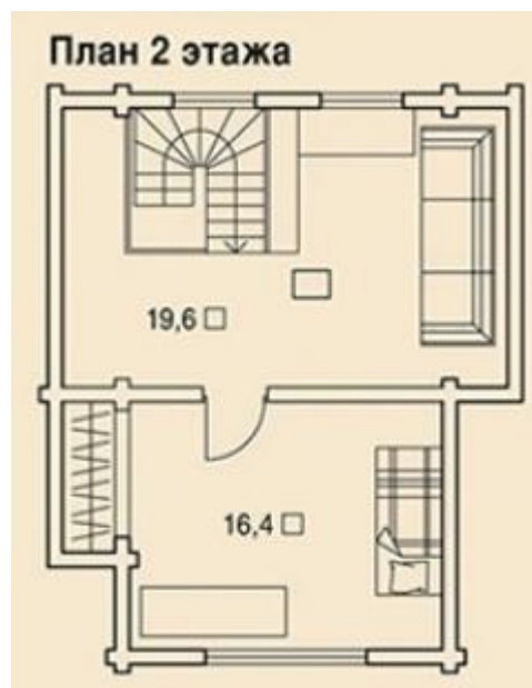
План мансардного этажа.
